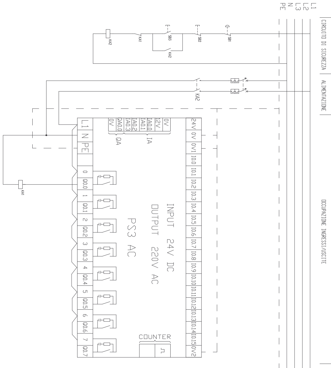
Figura 20 Esempio di alimentazione di un PLC rispettando criteri di sicurezza.
